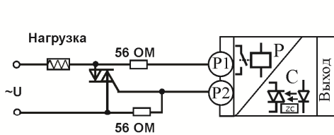
Подключение внешнего симистора
