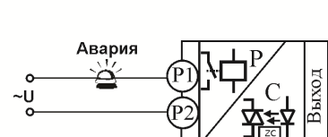
Подключение аварийной сигнализации
