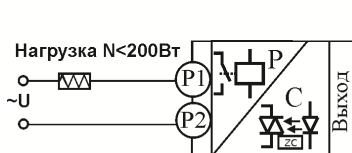
Подключение нагрузки менее 200 Вт
