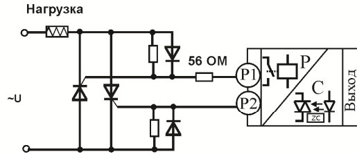
Подключение внешних тиристоров
