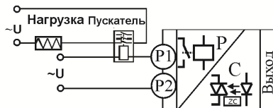
Подключение электромагнитного пускателя
