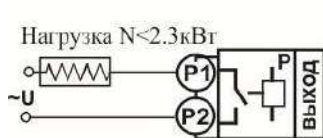
Подключение нагрузки менее 2,3 кВт
